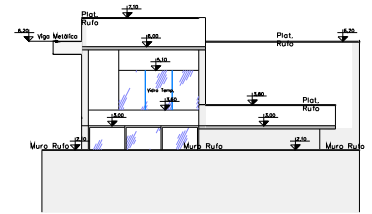
FACHADA POSTERIOR ESC. 1: 75
