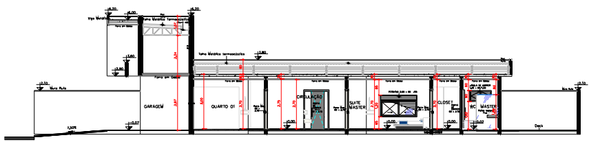
CORTE EE ESC. 1: 75
