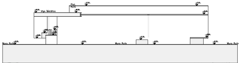
FACHADA LATERAL DIREITA ESC. 1: 75
