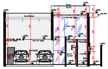
CORTE GG ESC. 1: 75
