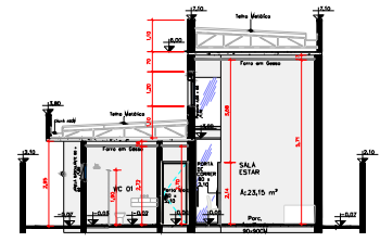
CORTE FF ESC. 1: 75
